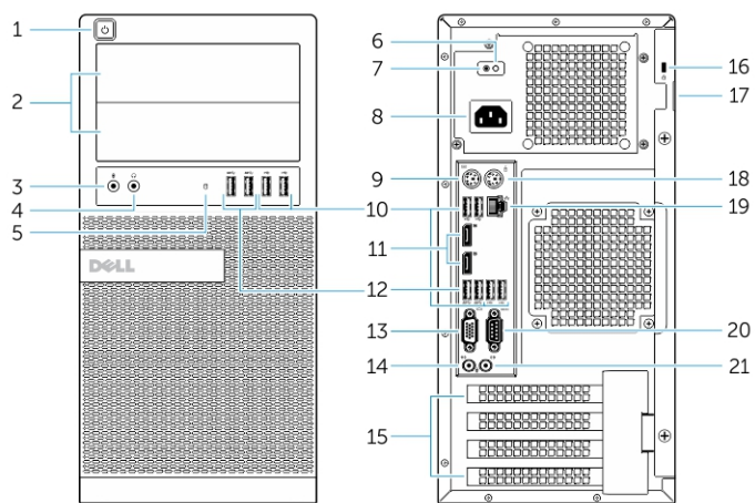
איור 1. מבט מלפנים ומבט מאחור על Mini Tower
